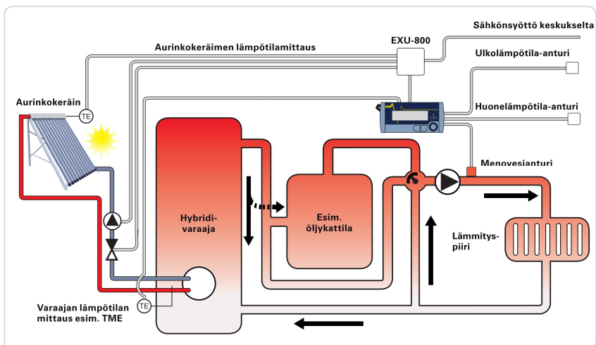
Periaatekuva hybridilämmityksestä, jossa lämmönsäädin ohjaa aurinkokeräimen ja varaajan välistä latauspumpua ja -venttiiliä sekä toimii lämmitysjärjestelmän säätimenä ulkolämpötilan ja menoveden lämpötilan perusteella.
