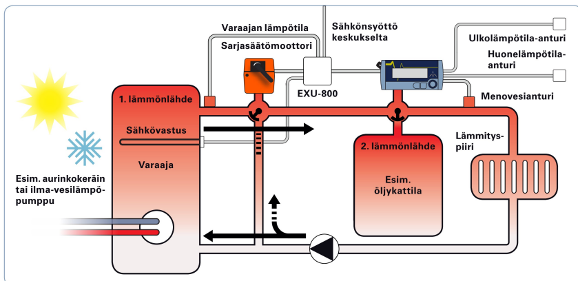
Periaatekuva hybridilämmityksestä, jossa sarjasäätömoottori ottaa tehoa 1. lämmönlähteestä. Kun 1. lämmönlähteestä loppuu teho, säädin alkaa ottaa lisätehoa 2. lämmönlähteestä. Pintalämpötila-anturi on kytketty mittaamaan (1. lämmönlähteen) varaajan lämpötilaa.
