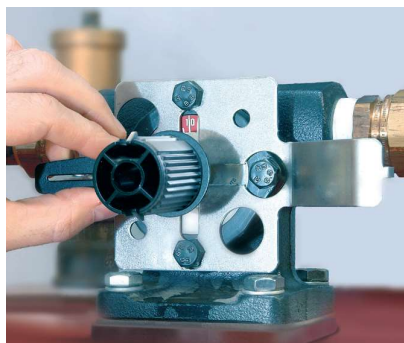
Irrota säätönuppi venttiilistä ja laita asennussarja paikoilleen. Paina EH-800 paikoilleen, kytke anturit ja käyttöjännite pistokeliittimiin, niin laite on käyttövalmis!
