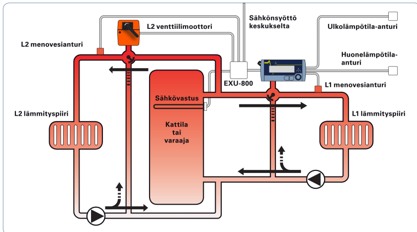
Periaatekuva kahden lämmityspiirin kytkennästä. Säädin ohjaa kumpaakin lämmityspiiriä saman ulkolämpötilatiedon, mutta eri menovesilämpötilatiedon perusteella. Kummallekin lämmityspiirille on oma säätökäyrä ja muut säätöön vaikuttavat asetukset.
